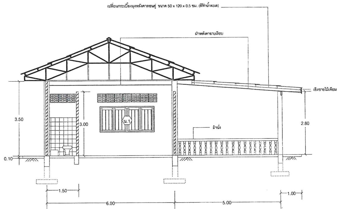
รูปตัด A-A Scale: 1 : 75
