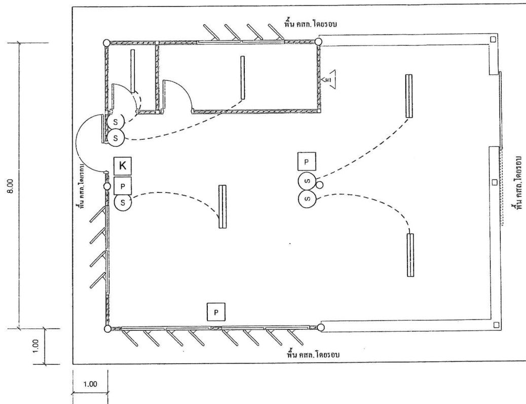
แปลนไฟฟ้าใหม่ Scale: 1 : 75
