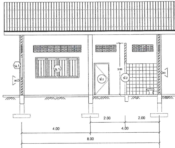
รูปตัด A-B Scale: 1 : 75
