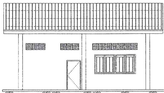
รูปด้าน 3 Scale: 1 : 100
